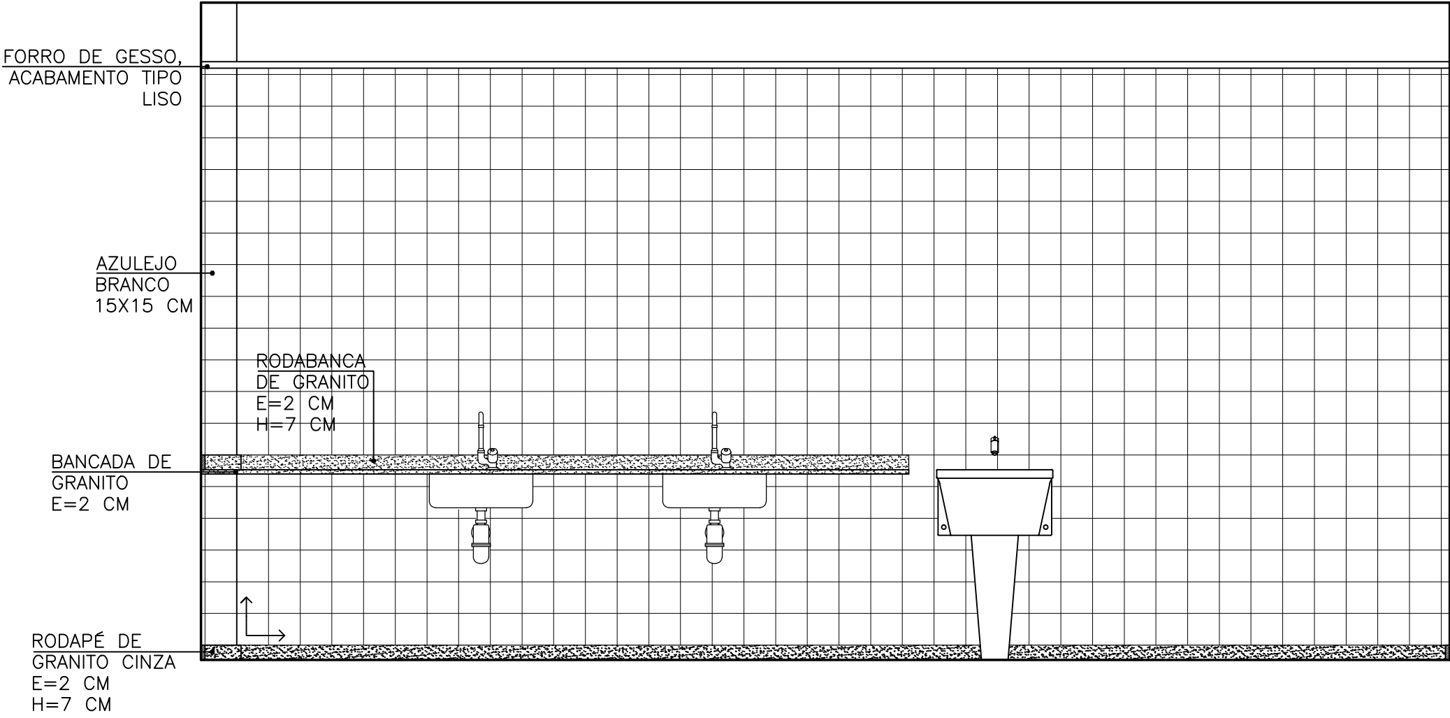
VISTA 03 ESC. 1/25
