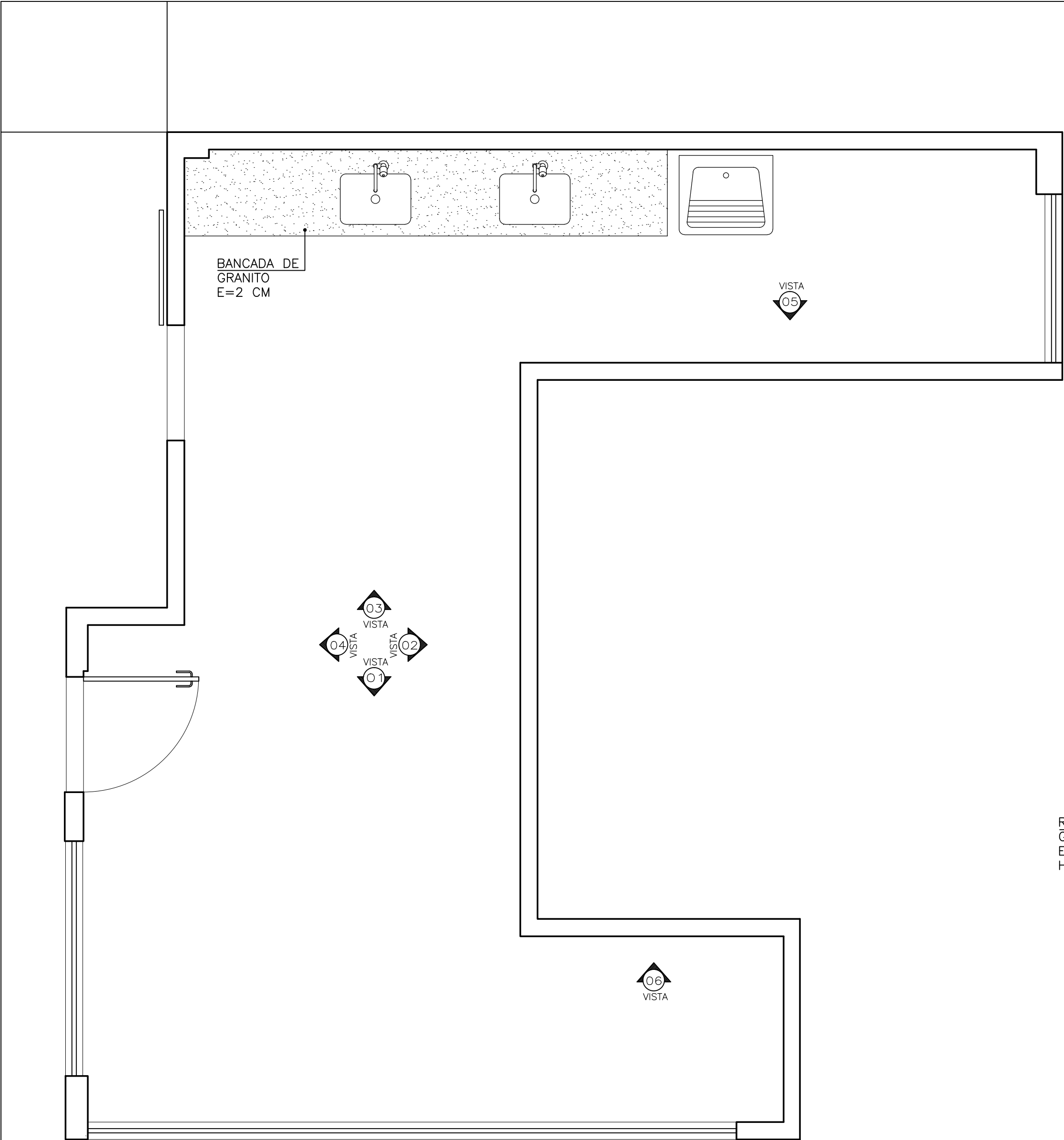
PLANTA BAIXA ESC. 1/25
