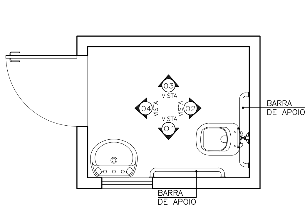
P PLANTA BAIXA ESC. 1/25
