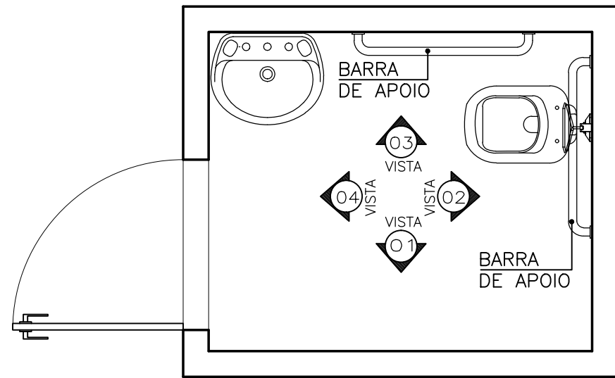
PLANTA BAIXA ESC. 1/25
