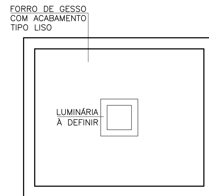
P PLANTA BAIXA - GESSO/ILUMINAÇÃO ESC. 1/25
