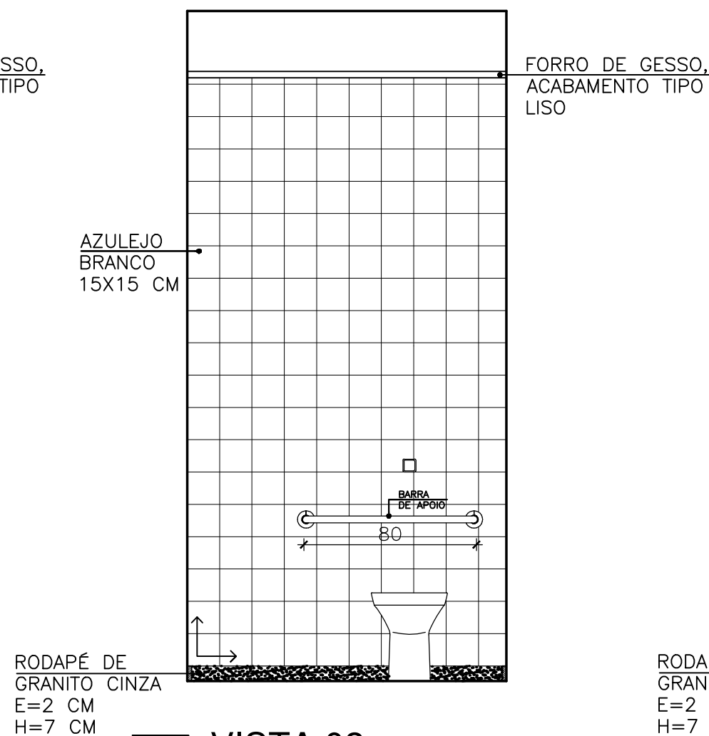
P VISTA 02 ESC. 1/25
