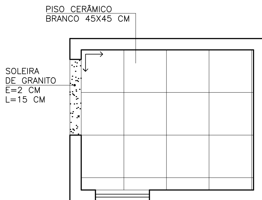
P PLANTA BAIXA - PAG. DE PISO ESC. 1/25
