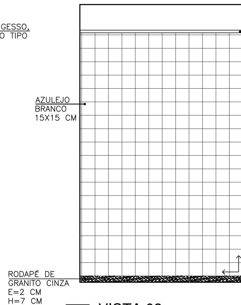
P VISTA 03 ESC. 1/25
