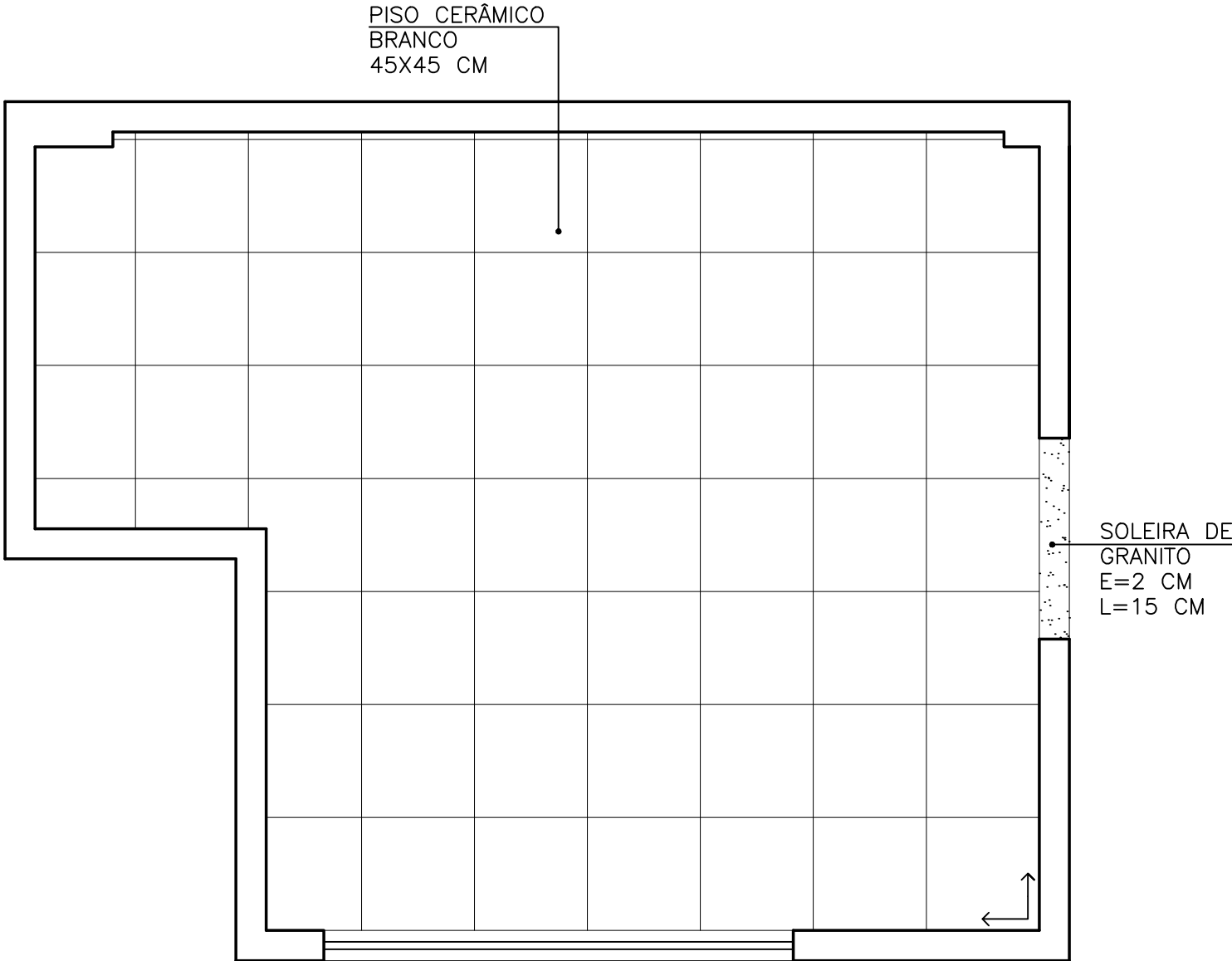
PLANTA BAIXA - PAG. DE PISO ESC. 1/25
