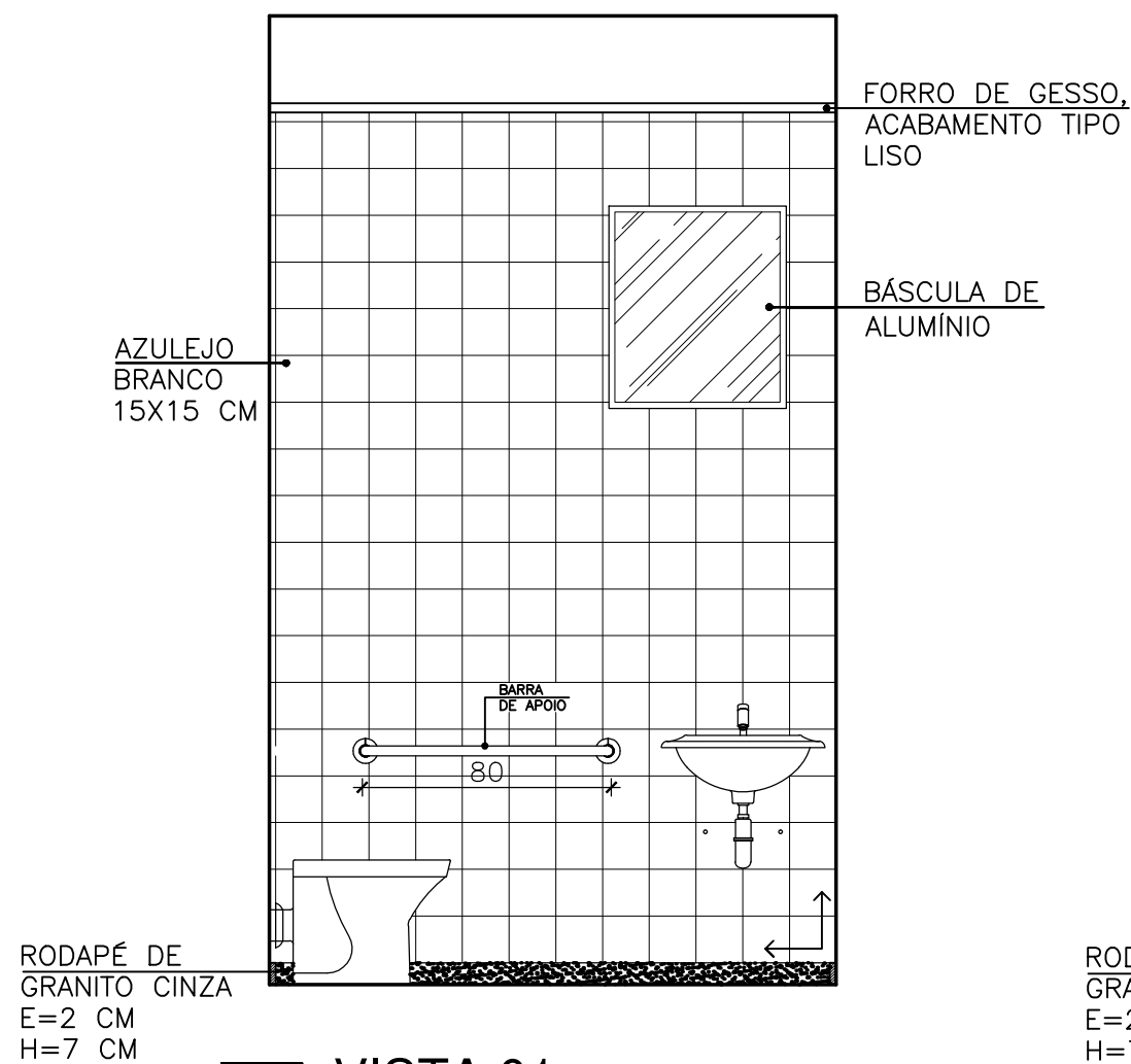
P VISTA 01 ESC. 1/25
