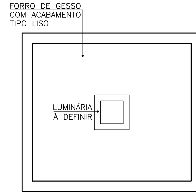
P PLANTA BAIXA - GESSO/ILUMINAÇÃO ESC. 1/25
