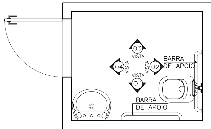
P PLANTA BAIXA ESC. 1/25
