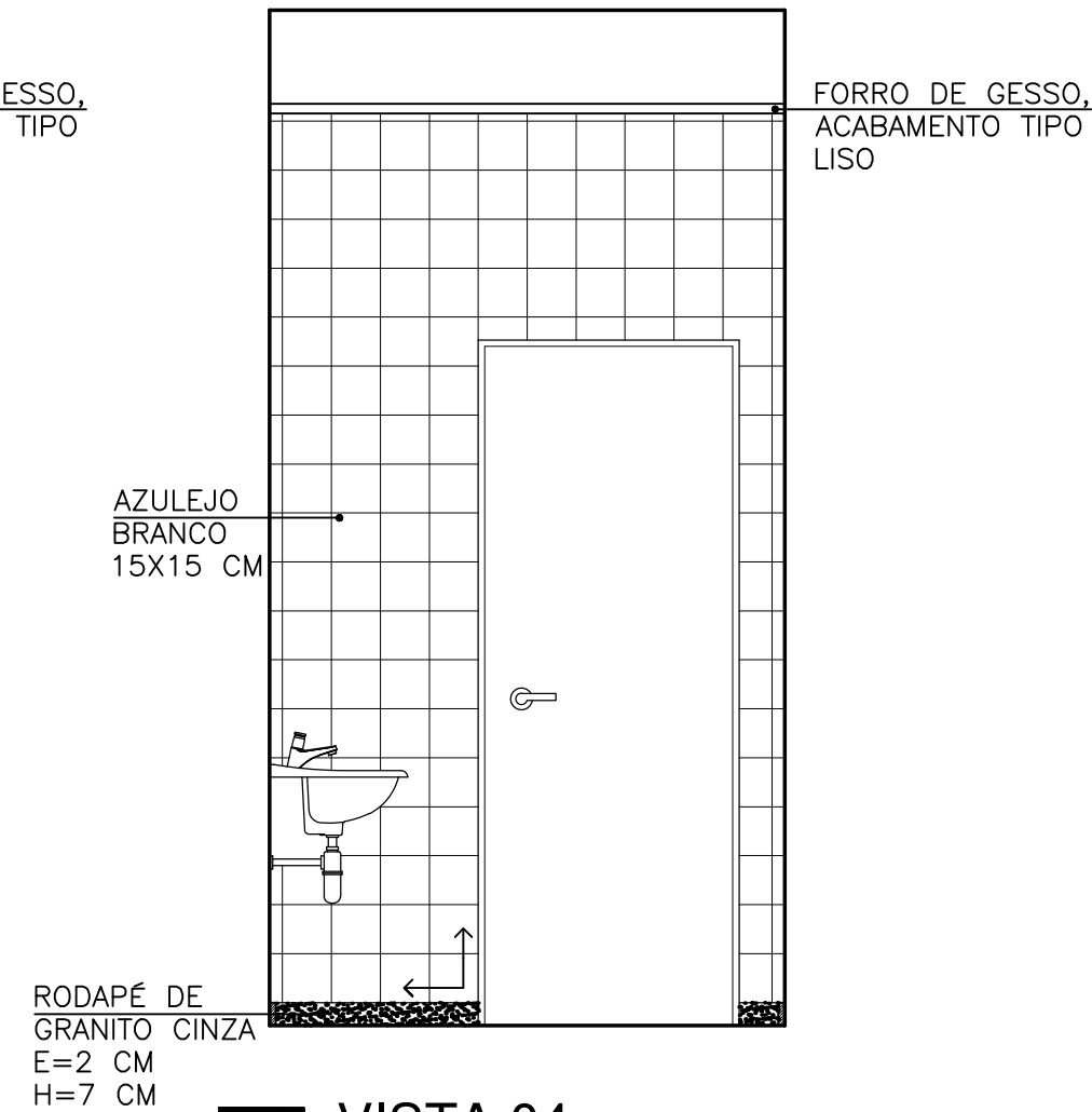
P VISTA 04 ESC. 1/25
