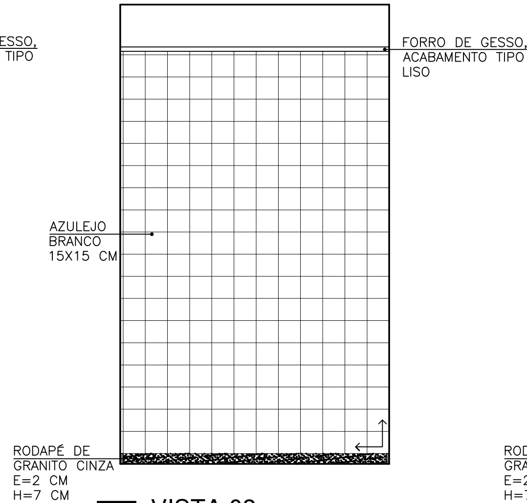
P VISTA 03 ESC. 1/25
