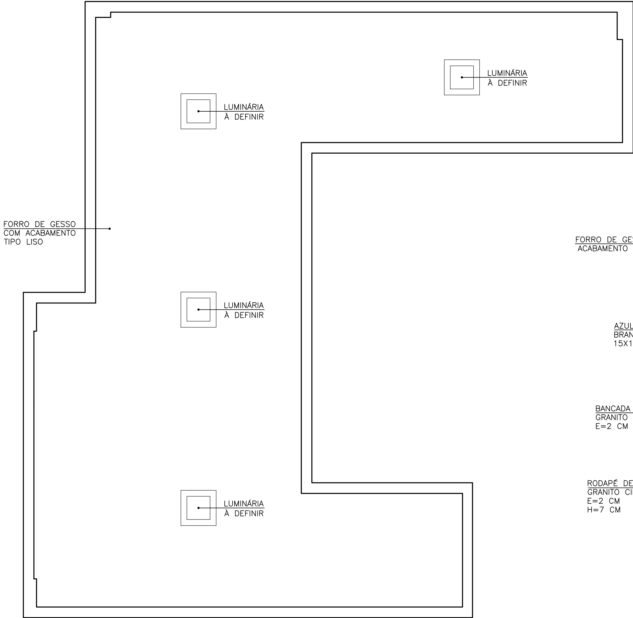
PLANTA BAIXA - GESSO/ILUMINAÇÃO ESC. 1/25
