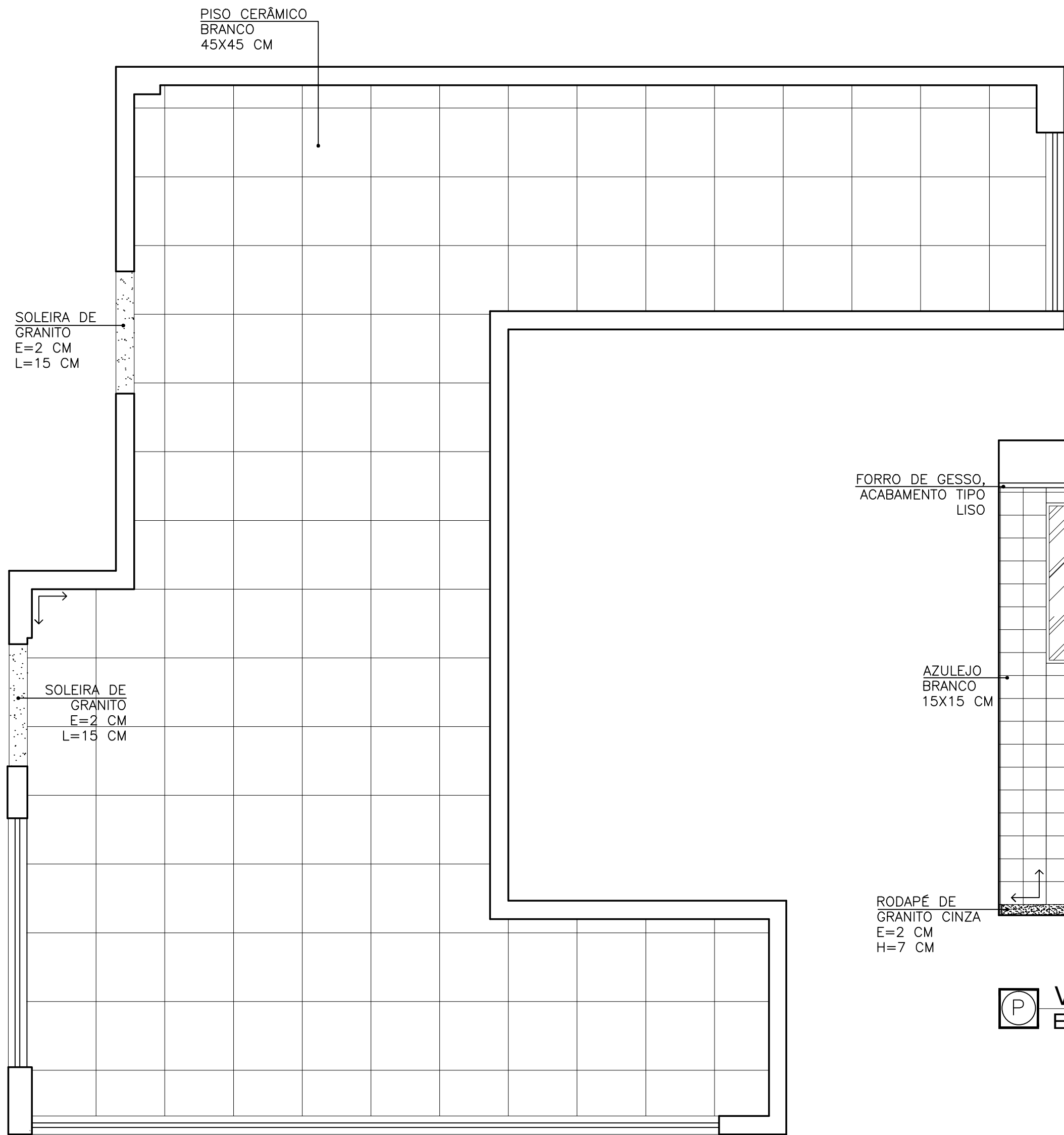
PLANTA BAIXA - PAG. DE PISO ESC. 1/25
