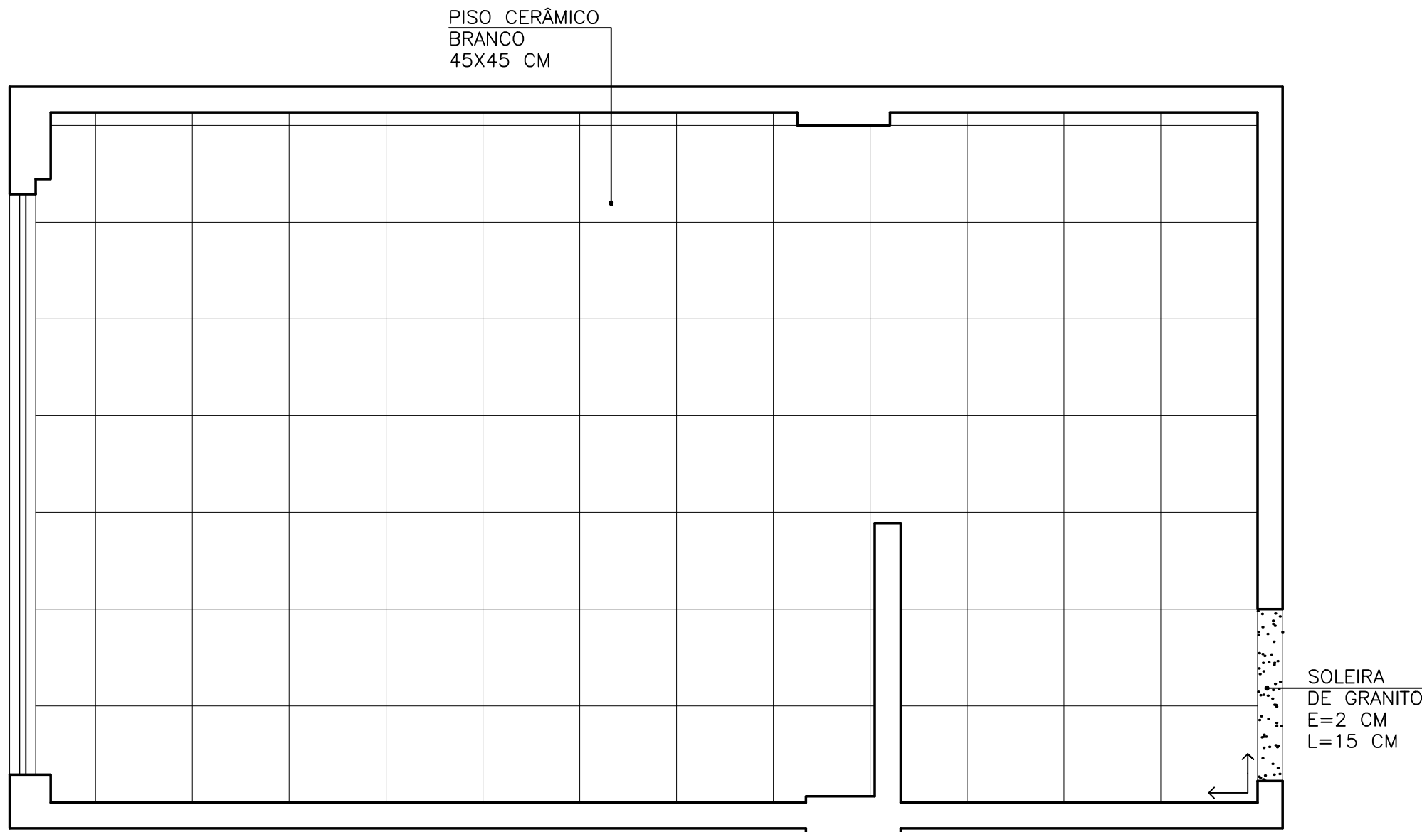
PLANTA BAIXA - PAG. DE PISO ESC. 1/25
