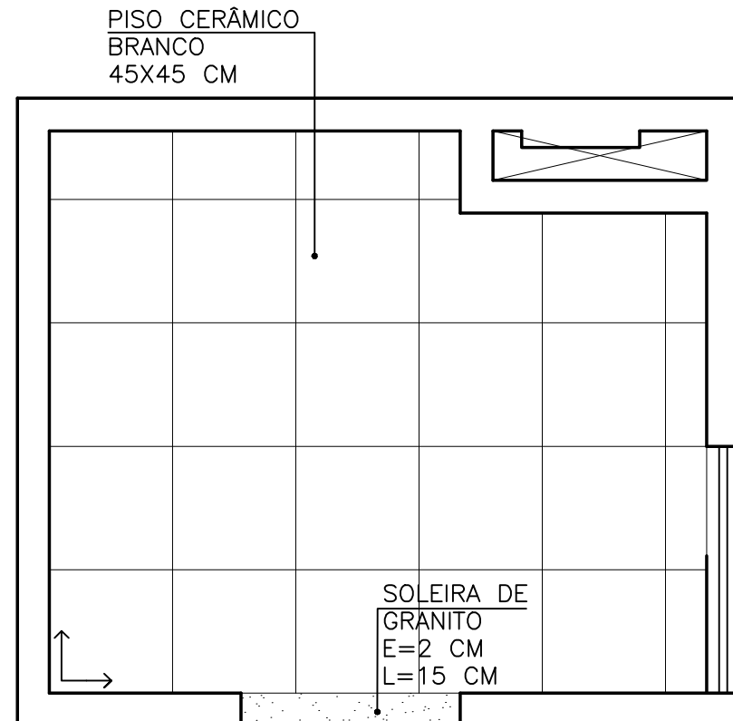
P PLANTA BAIXA - PAG. DE PISO ESC. 1/25
