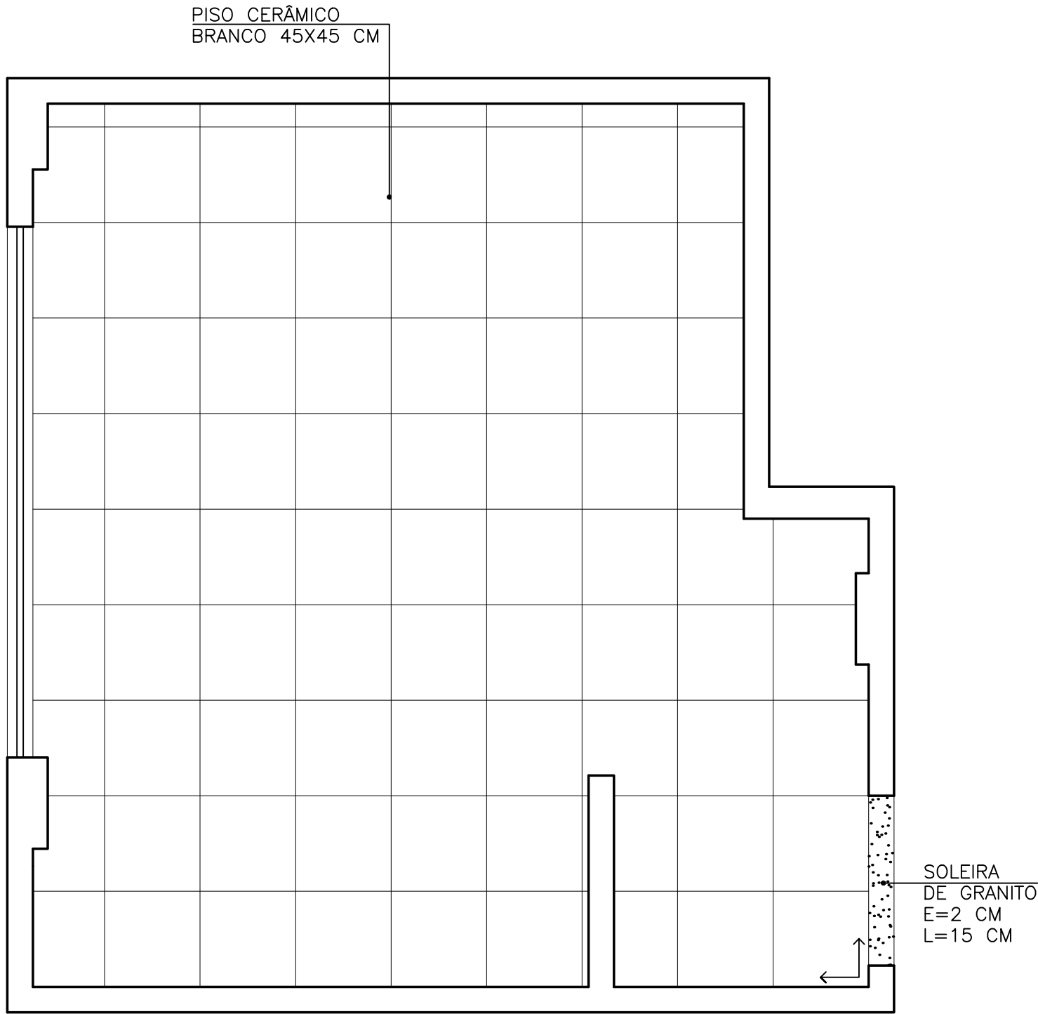
P PLANTA BAIXA - PAG. DE PISO ESC. 1/25
