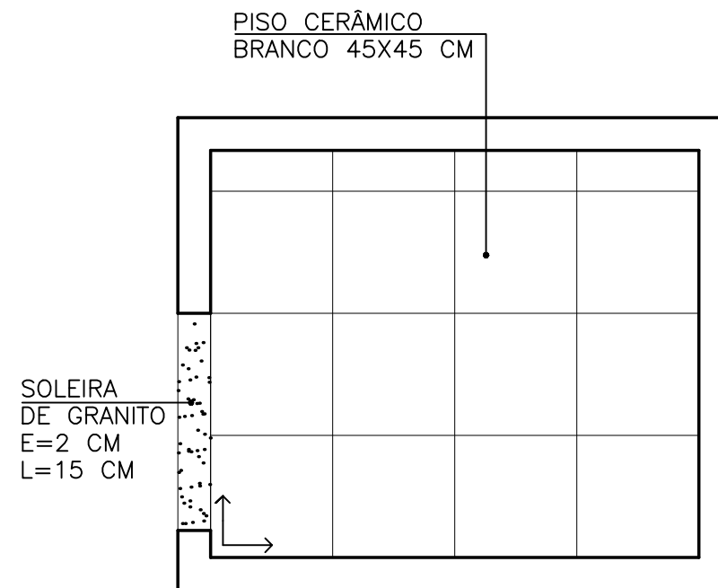
PLANTA BAIXA - PAG. DE PISO ESC. 1/25
