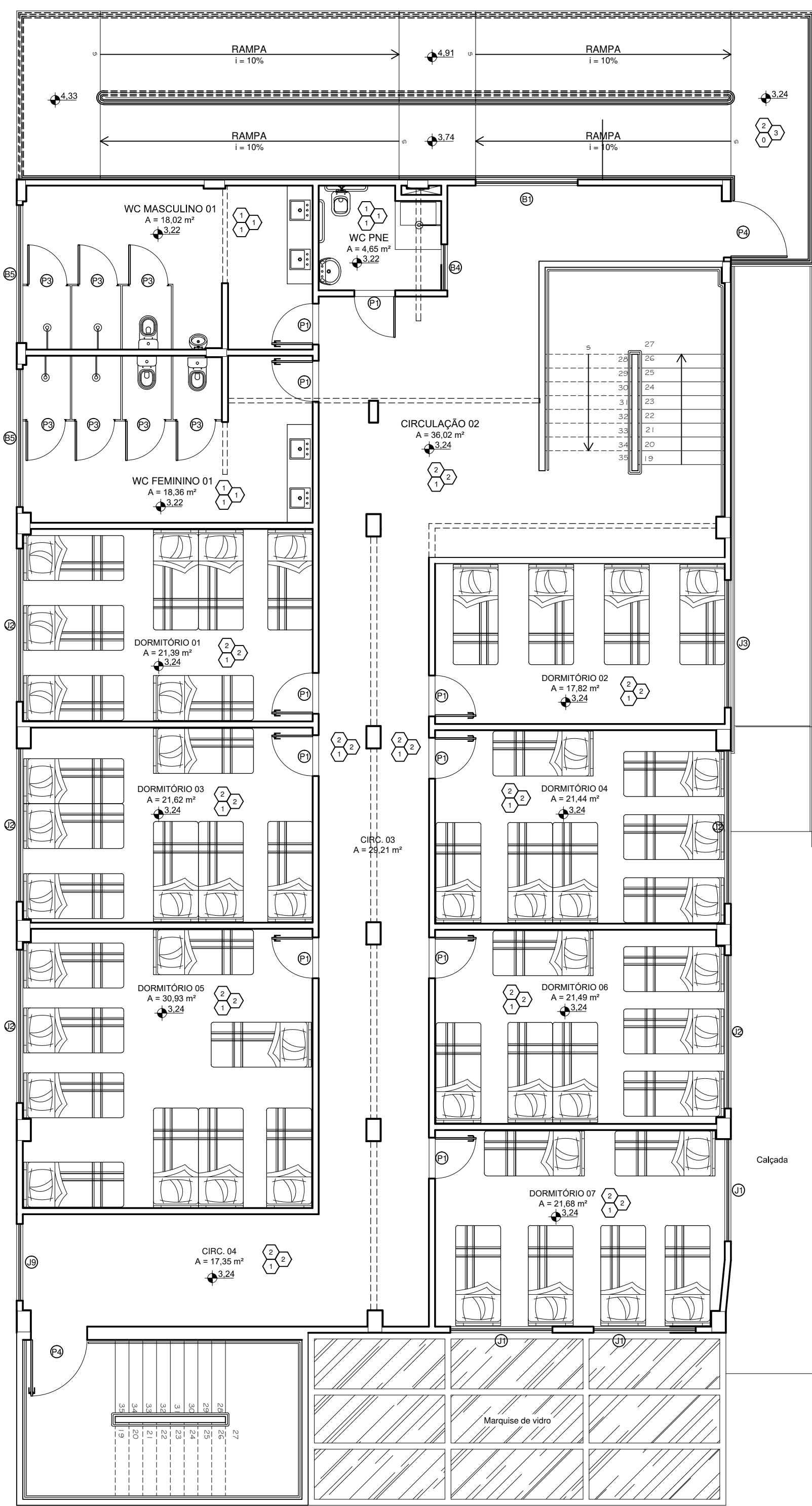
PLANTA BAIXA - 1º PAV. ESC. 1 / 75
