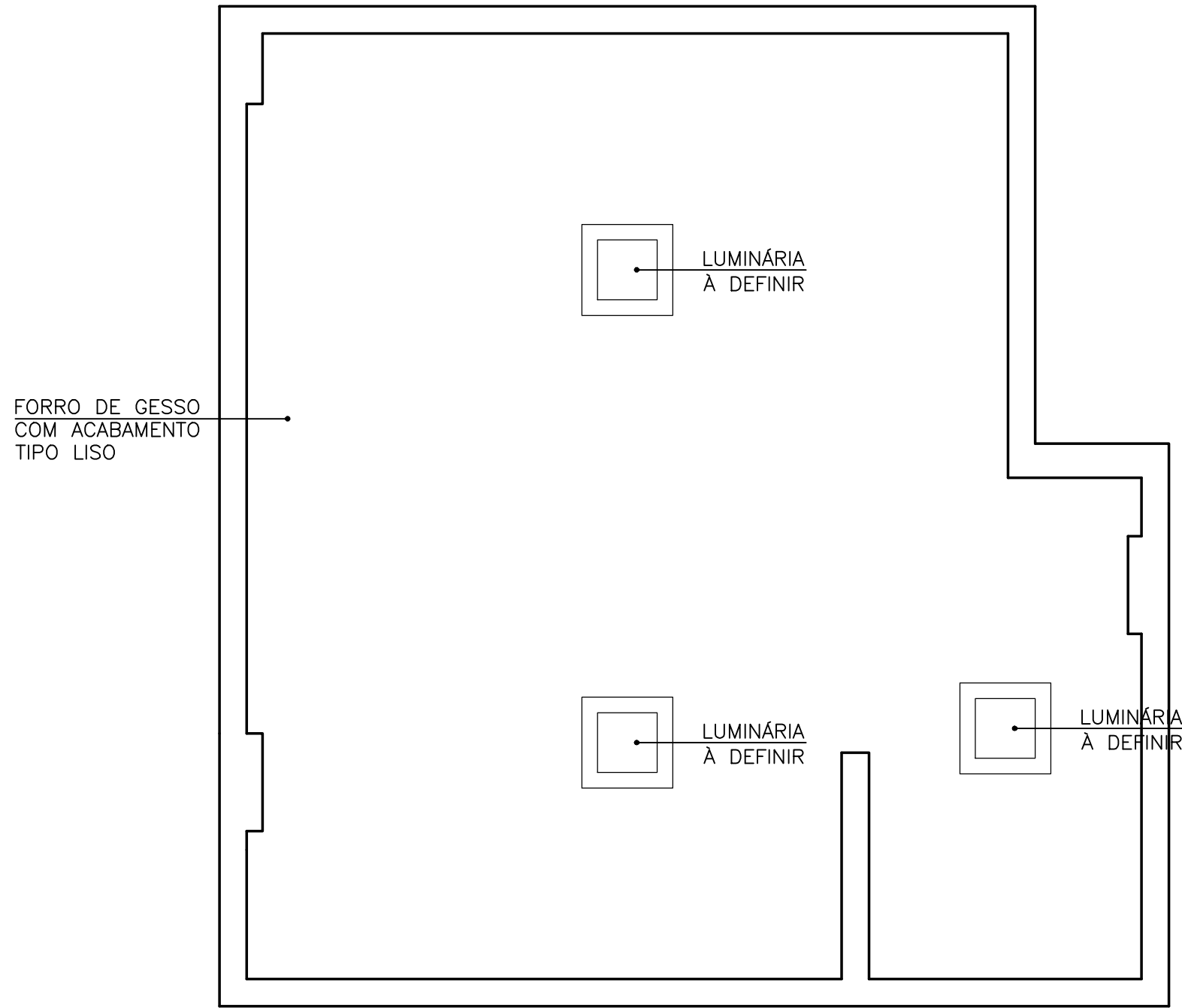
P PLANTA BAIXA - PAG. DE PISO ESC. 1/25
