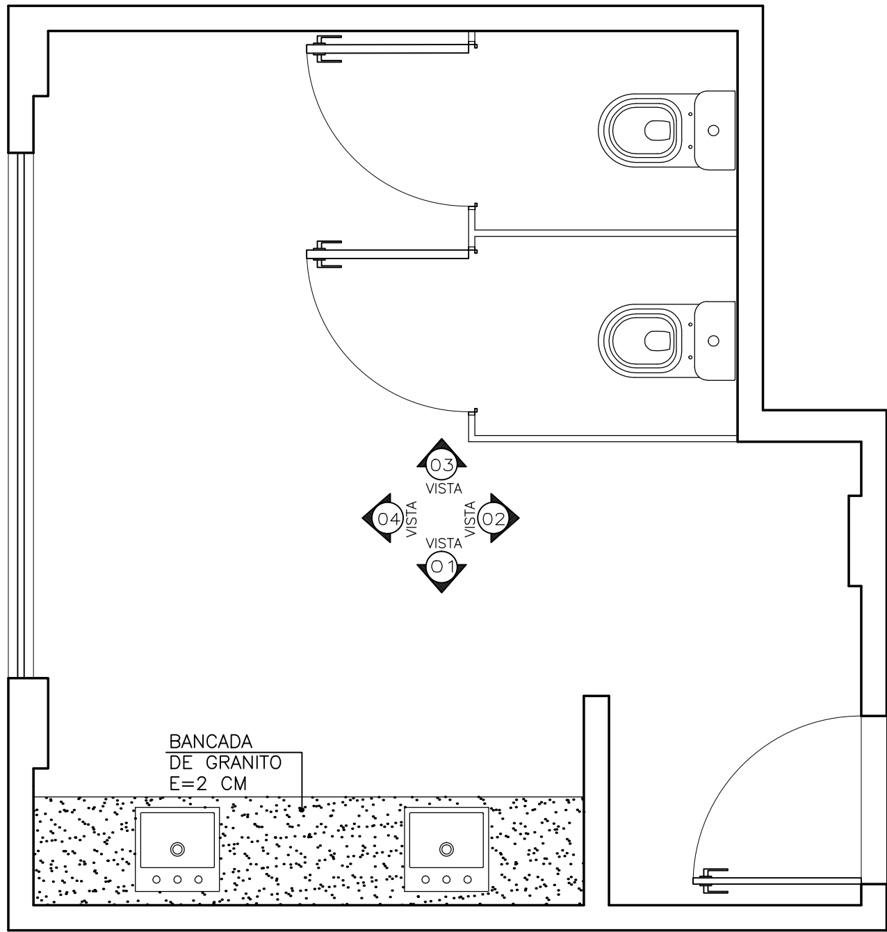
P PLANTA BAIXA ESC. 1/25
