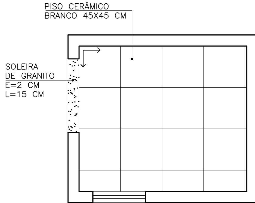
P PLANTA BAIXA - PAG. DE PISO ESC. 1/25
