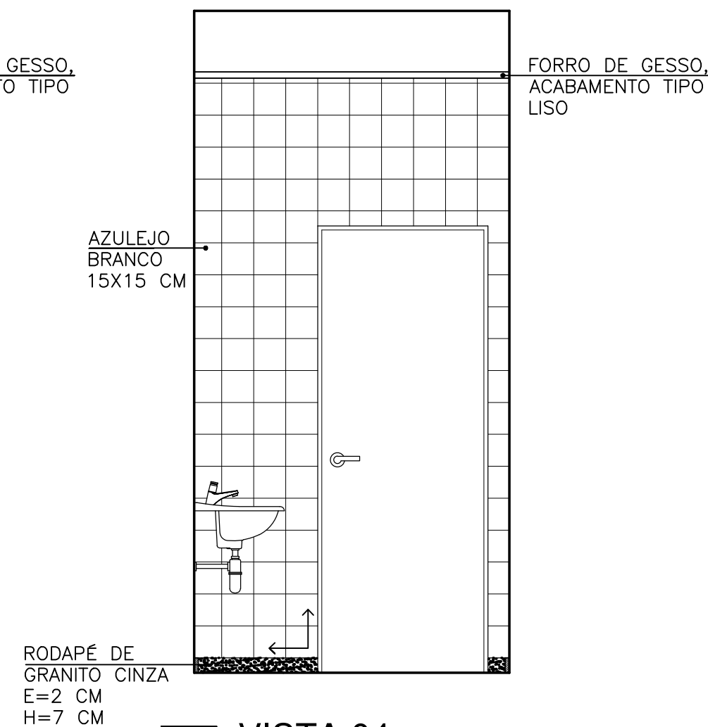
P VISTA 04 ESC. 1/25
