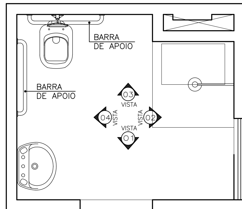
P PLANTA BAIXA ESC. 1/25
