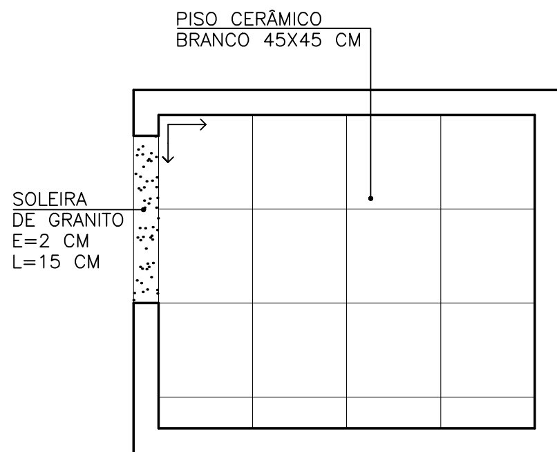
P PLANTA BAIXA - PAG. DE PISO ESC. 1/25
