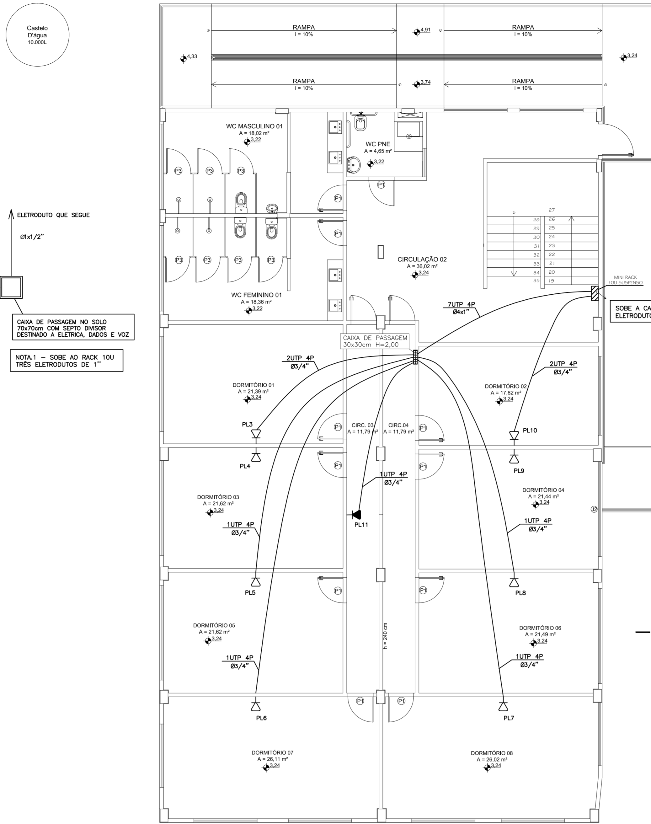
Planta Baixa - 1º Pav. ESC. 1 / 75
