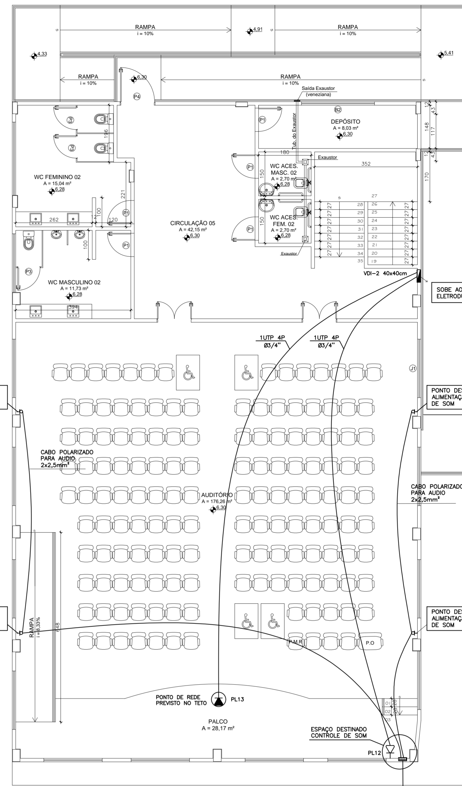
Planta Baixa - 2º Pav. ESC. 1 / 75
