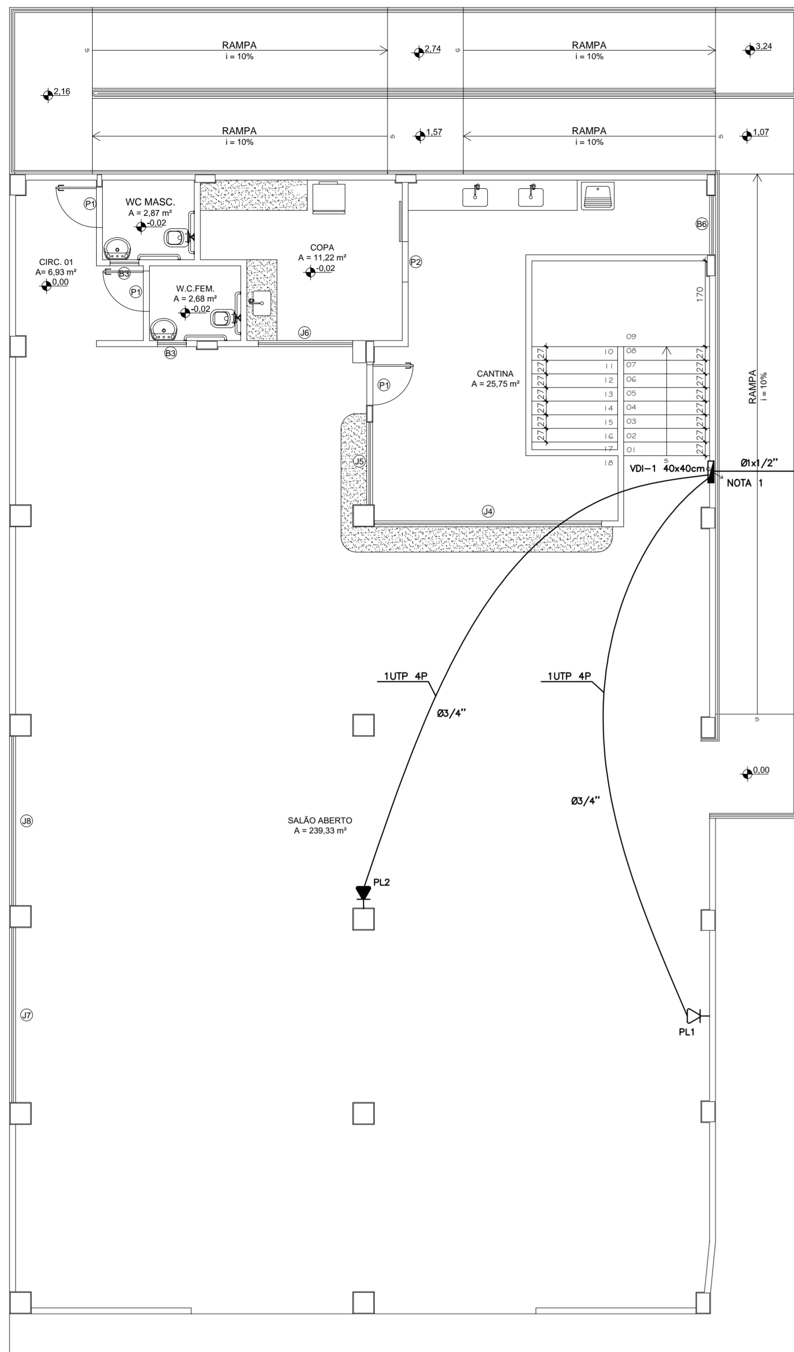
Planta Baixa - Térreo ESC. 1 / 75
