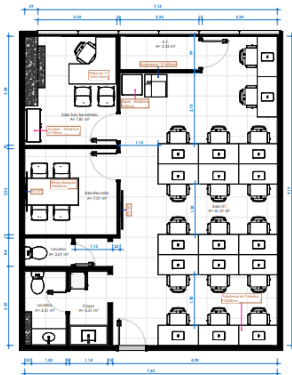
1 PLANTA DE LAYOUT - BANCO MUNDIAL 1 : 50
